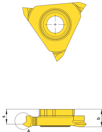
Abbildung zeigt / Drawing shows: TE3.NP18.02 M R
