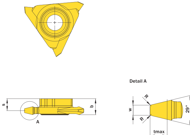
Abbildung zeigt / Drawing shows: TE3.AC06.01 MR
