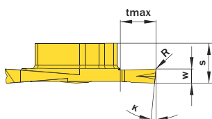
Abbildung zeigt / Drawing shows: TE3.L200.05 PT L
